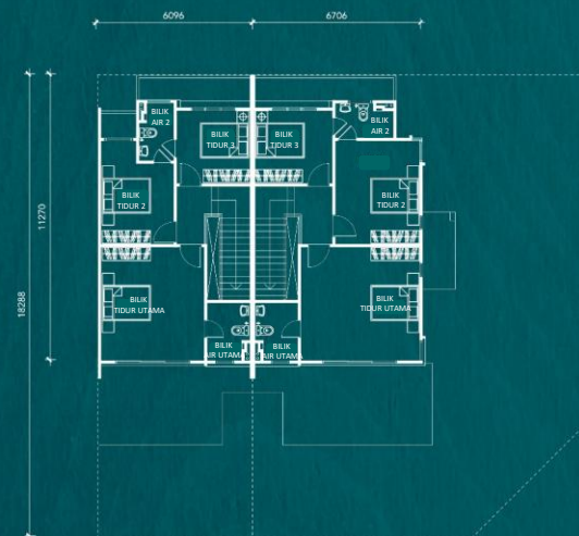
Tingkat Satu
