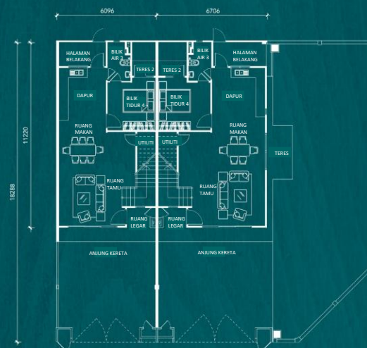
Tingkat Bawah
