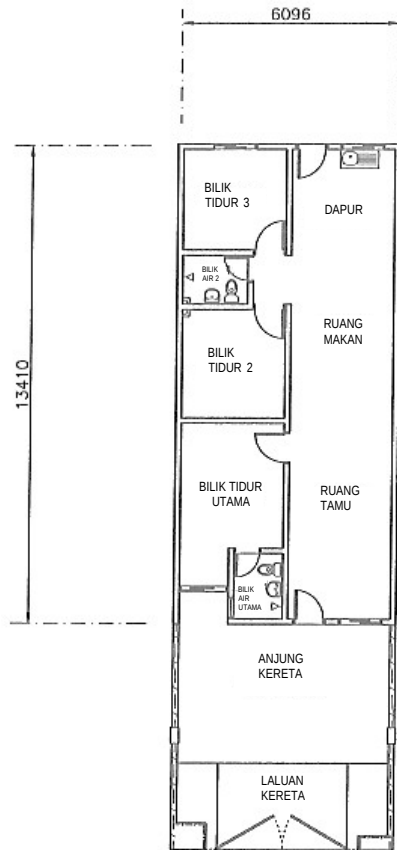
PELAN LANTAI TINGKAT BAWAH
