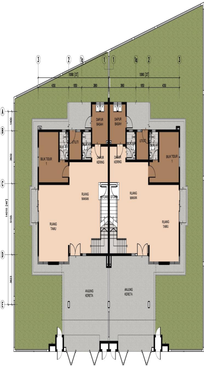
RUMAH SEMI-D - JENIS C PELAN LANTAI Skala 1:125
