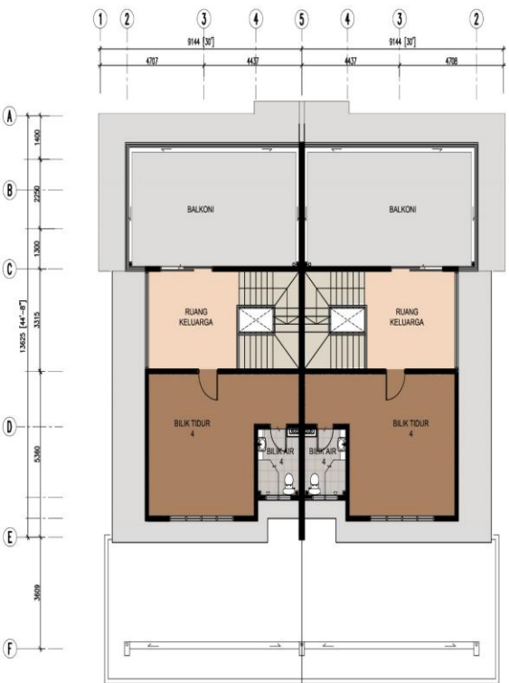
RUMAH SEMI-D - JENIS B PELAN LANTAI TINGKAT 2
