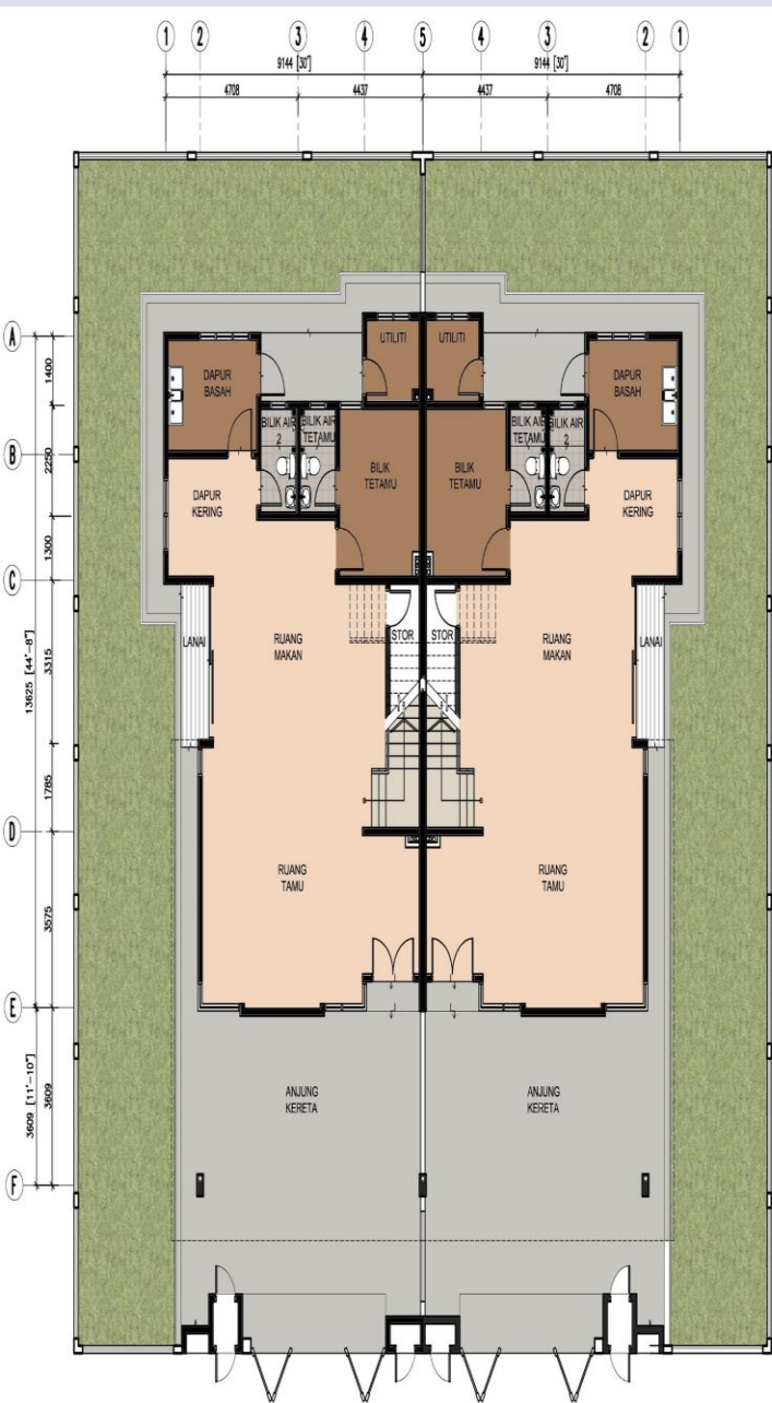
RUMAH SEMI-D - JENIS A PELAN LANTAI
