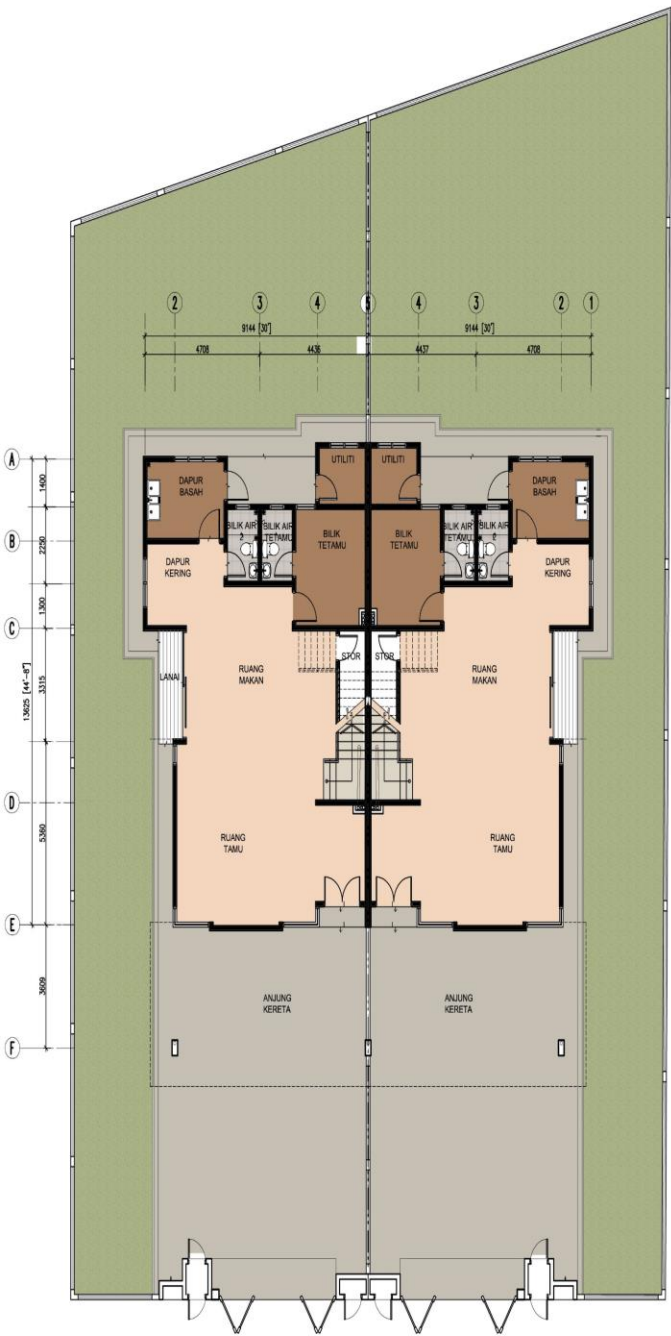
RUMAH SEMI-D - JENIS B PELAN LANTAI
