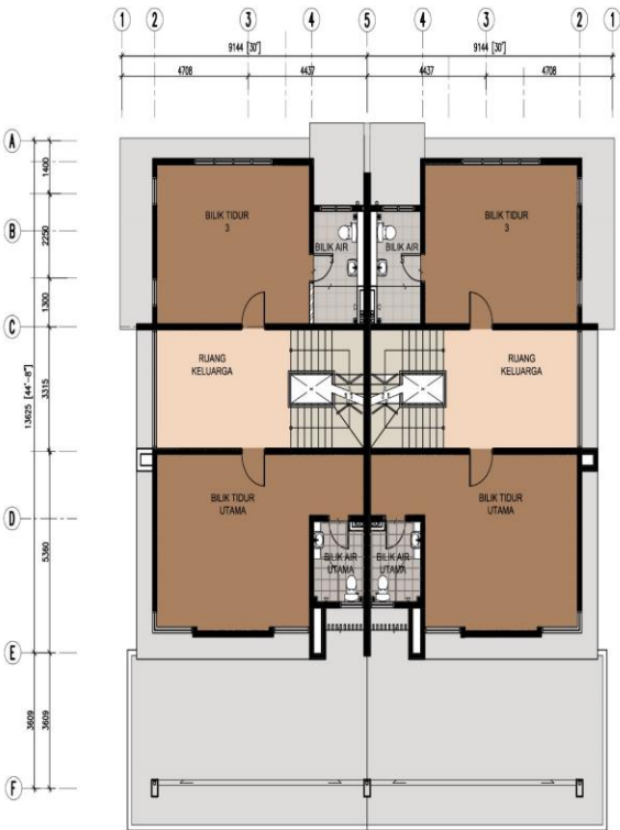
RUMAH SEMI-D - JENIS B PELAN LANTAI TINGKAT 1
