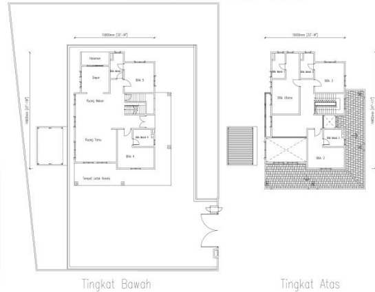
Pelan Lantai Rumah Banglo 2 Tingkat - Jenis B
