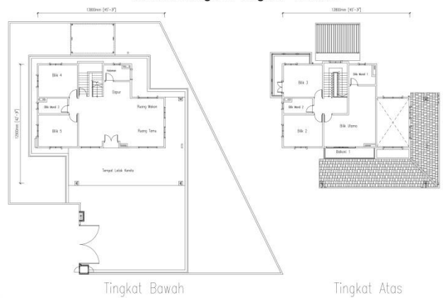
Pelan Lantai Rumah Banglo 2 Tingkat - Jenis D
