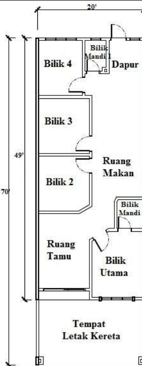
Rumah Teres 1 Tingkat
