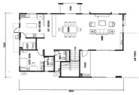
RUMAH BANGLO 2 TINGKAT - PELAN TINGKAT BAWAH
