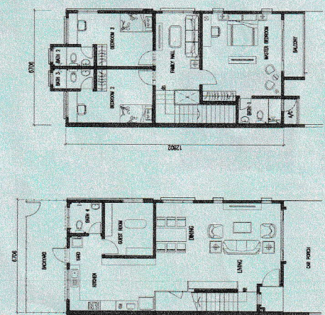
RUMAH TERES 2 TINGKAT - PELAN TINGKAT BAWAH
