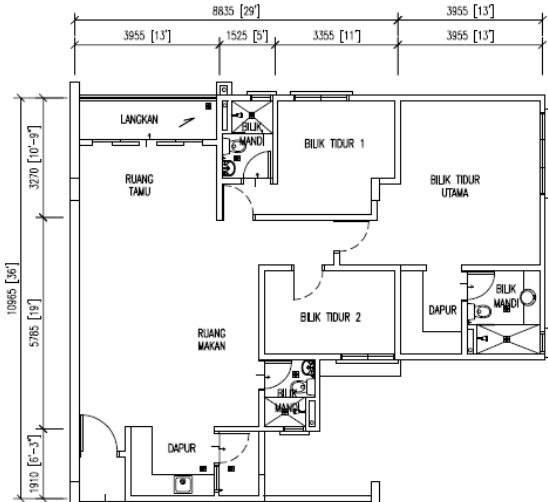
TYPE C4 3 Bilik 1,220 sq.ft
