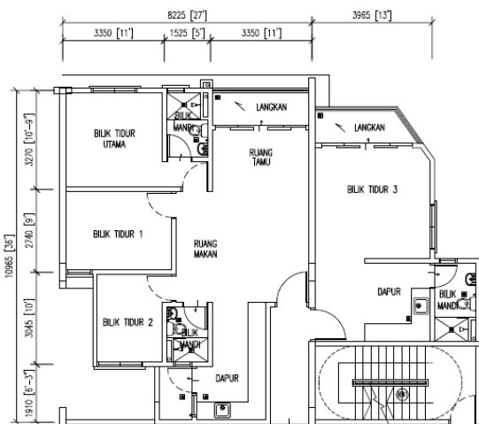
TYPE B1 4 Bilik 1,238 sq.ft
