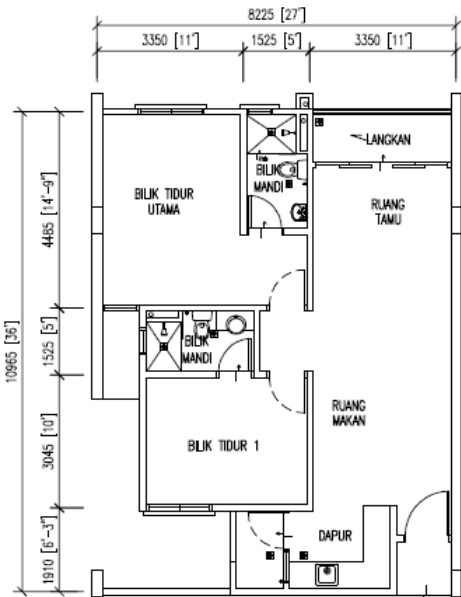
TYPE C2 2 Bilik 855 sq.ft
