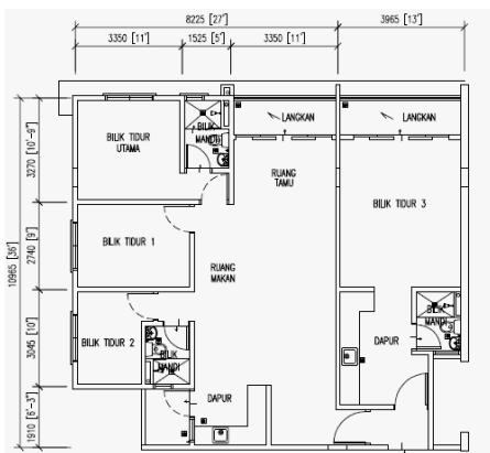
TYPE B3 4 Bilik 1,352 sq.ft
