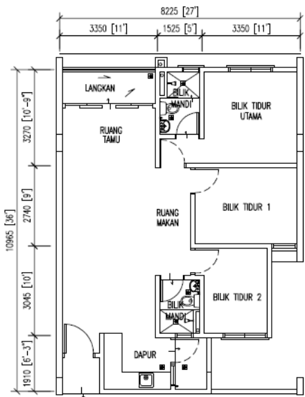
TYPE A 3 Bilik 872 sq.ft
