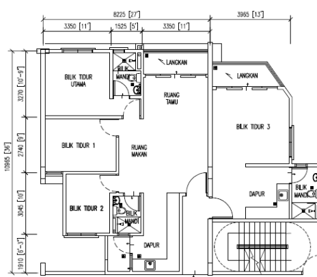
TYPE C6 4 Bilik 1,238 sq.ft
