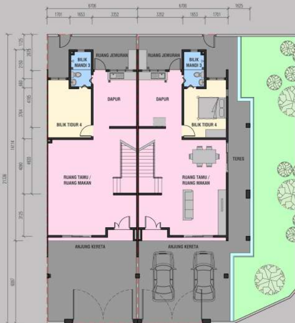
PELAN LANTAI 1
