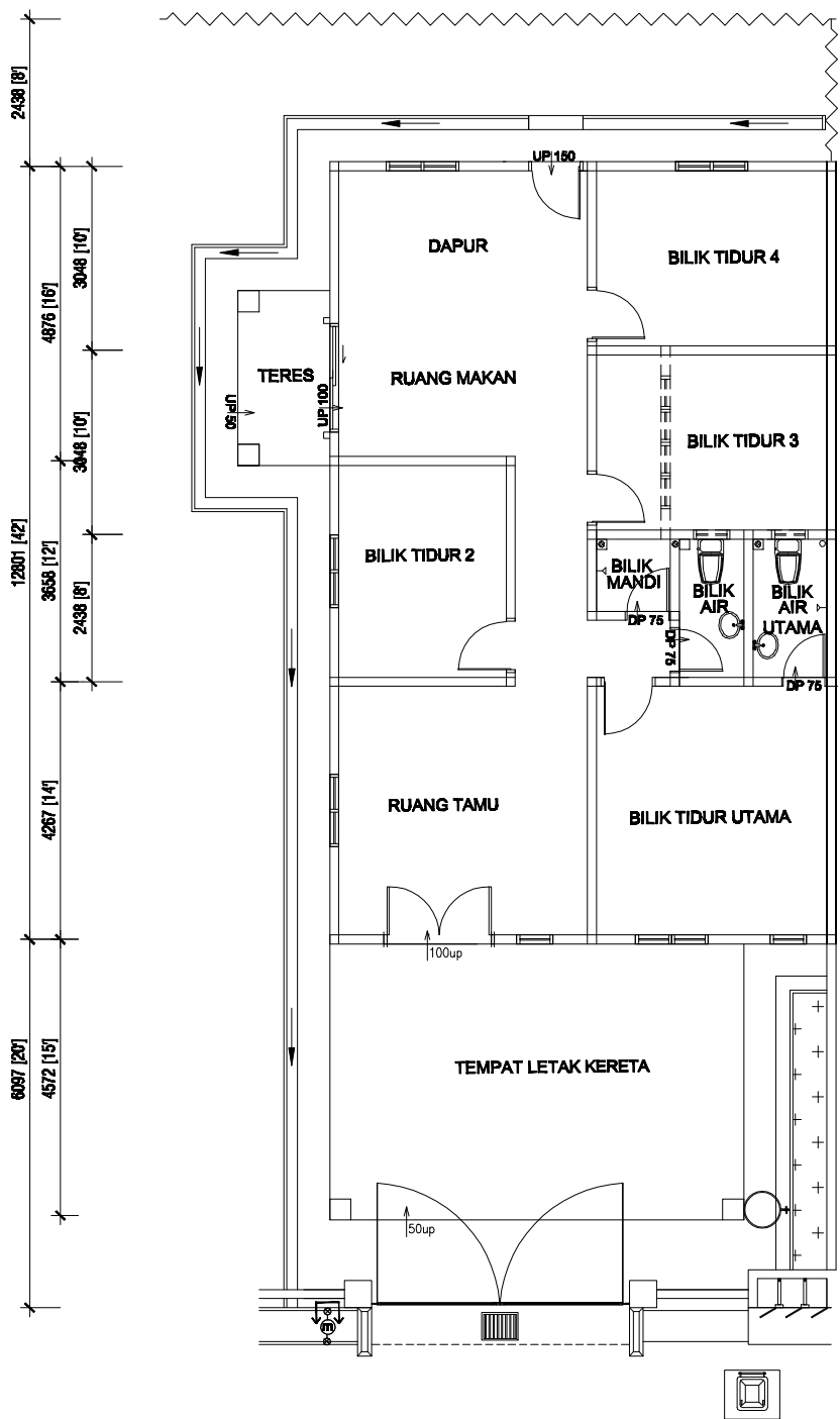
PELAN LANTAI ( KIRI ) ( PTD 6596,PTD 6598,PTD 6600 )
