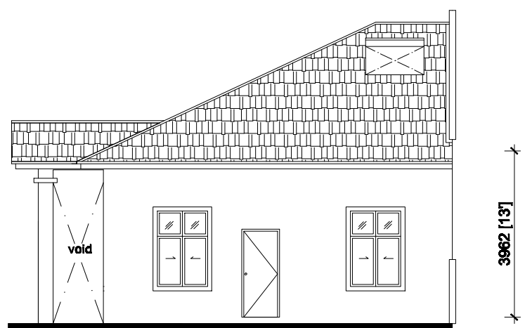
PANDANGAN BELAKANG ( PTD 6597,PTD 6599,PTD 6601 )
