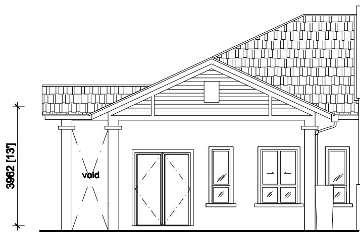
PANDANGAN HADAPAN ( PTD 6596,PTD 6598,PTD 6600 )
