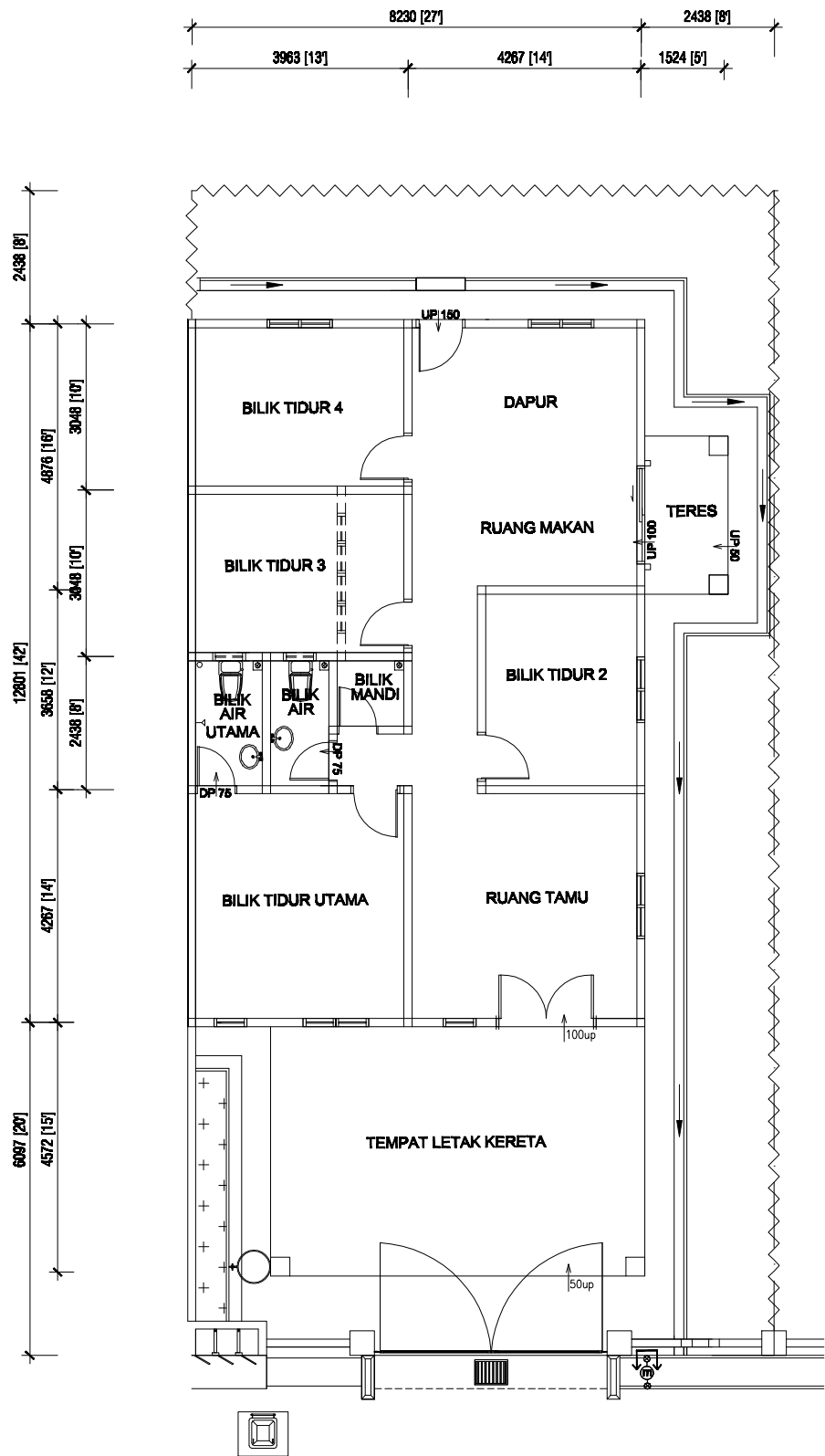
PELAN LANTAI ( KANAN ) ( PTD 6597,PTD 6599,PTD 6601 )
