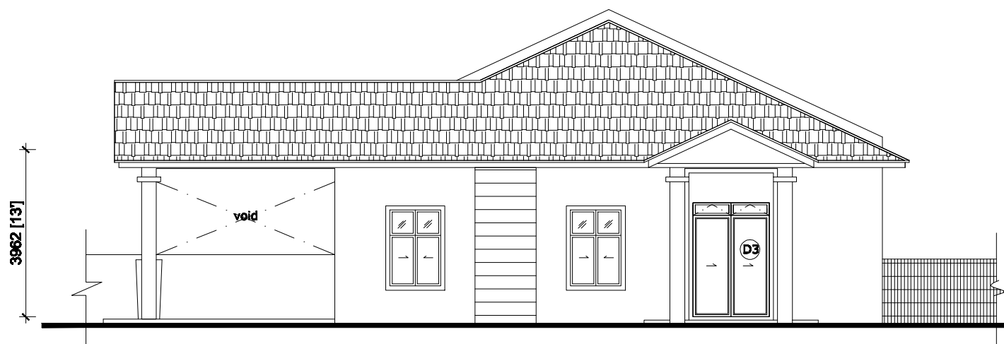
PANDANGAN SISI ( PTD 6597,PTD 6599,PTD 6601 )
