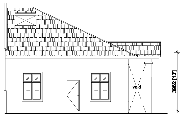
PANDANGAN BELAKANG ( PTD 6596,PTD 6598,PTD 6600 )
