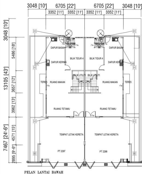
RUMAH BERKEMBAR 2 TINGKAT (JENIS B) (PT 2297 - 2299)
