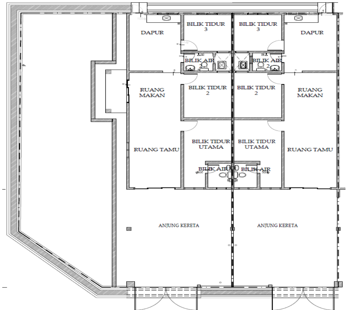
PELAN LANTAI (RUMAH TERES 1 TINGKAT)
