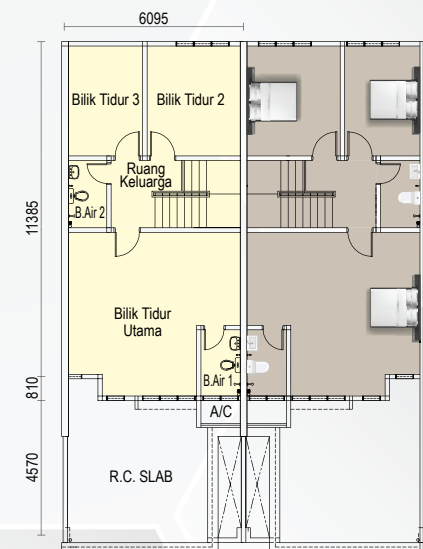
Tingkat Atas
