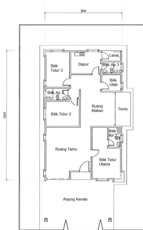
Pelan Lantai
