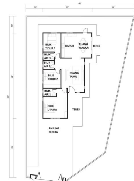
Rumah Sesebuah 1 Tingkat Jenis E – 1 Unit
