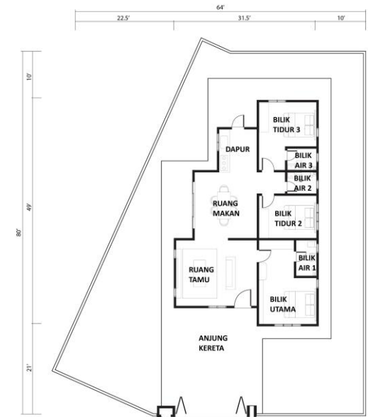
Rumah Sesebuah 1 Tingkat Jenis C – 2 Unit
