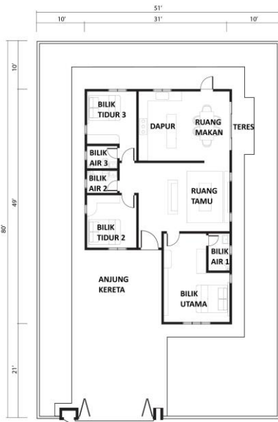
Pelan Lantai
