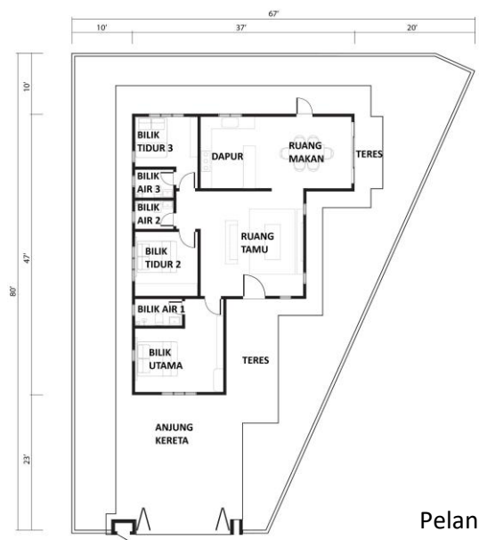
Rumah Sesebuah 1 Tingkat Jenis D – 1 Unit
