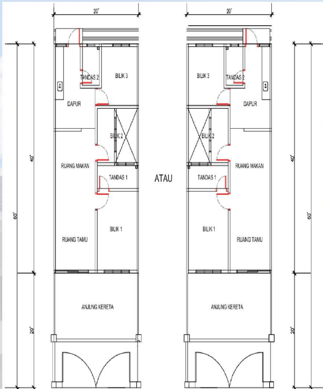
PELAN LANTAI (RUMAH TERES SATU TINGKAT 20' x 60') (LOT TENGAH)
