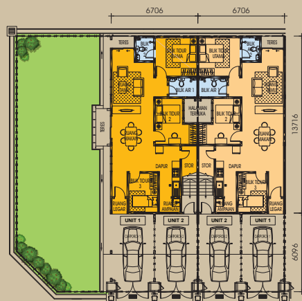
TINGKAT BAWAH - UNIT 1 (BLOK C & D)
