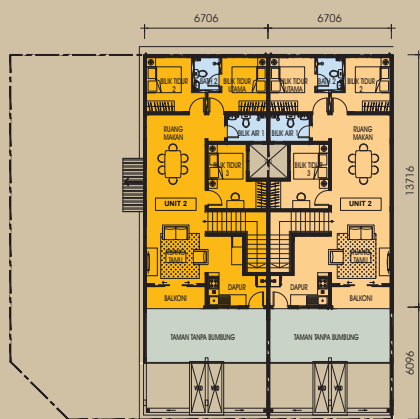
TINGKAT SATU - UNIT 2 (BLOK C & D)
