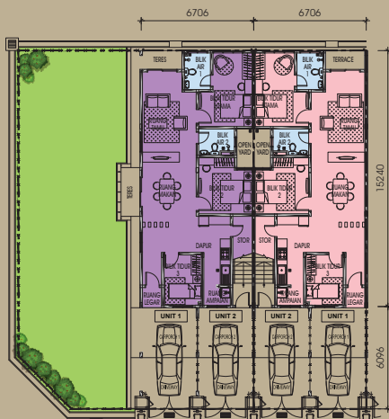
TINGKAT BAWAH - UNIT 1 (BLOK A & B)
