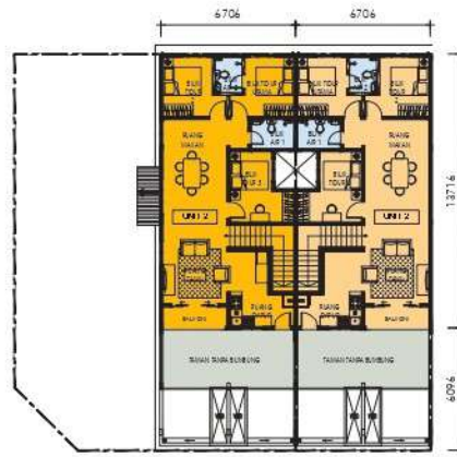
TINGKAT SATU - UNIT 2 (BLOK G & H)
