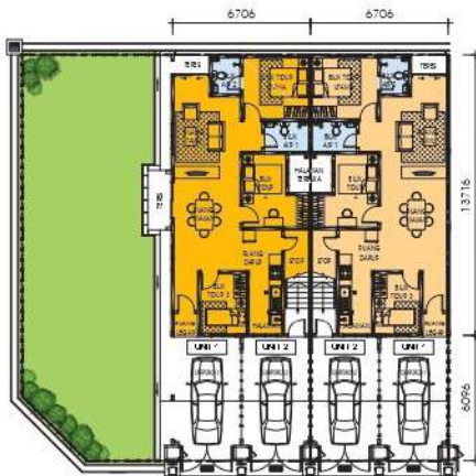
TINGKAT BAWAH - UNIT 1 (BLOK G & H)
