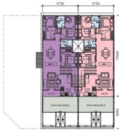
TINGKAT SATU - UNIT 2 (BLOK A, B, C, D, E & F)
