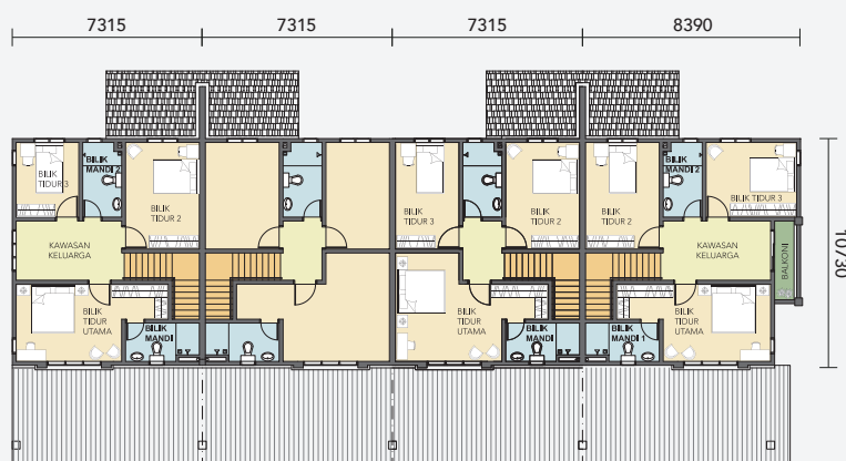
Pelan Lantai Aras Satu
