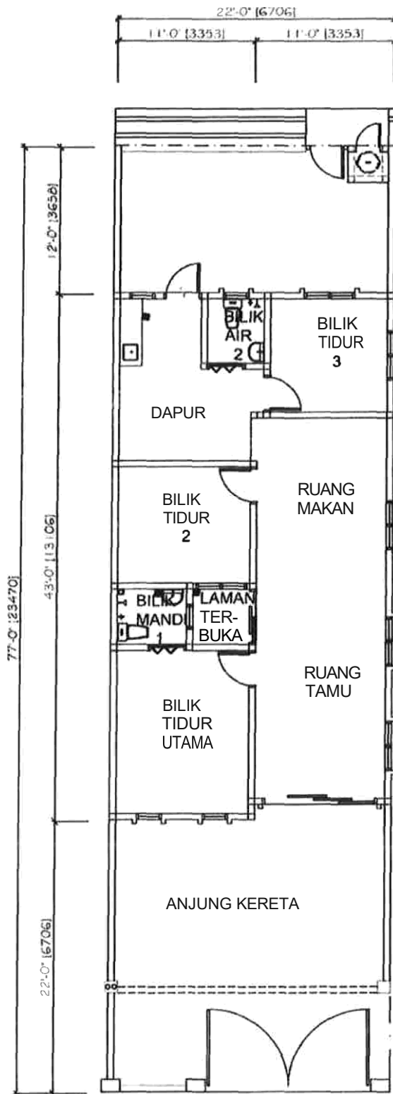
PELAN LANTAI
