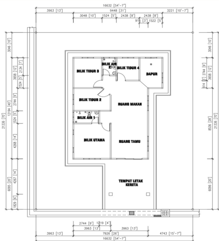
PELAN LANTAI
