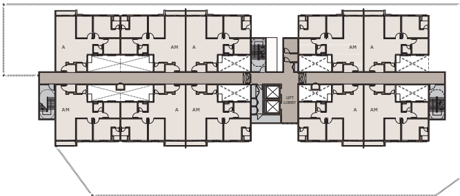
PELAN LANTAI TIPIKAL (TINGKAT 6 HINGGA TINGKAT 15)
