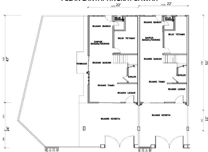
PELAN LANTAI TINGKAT BAWAH
