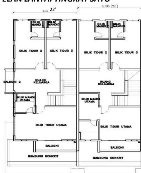
PELAN LANTAI TINGKAT SATU
