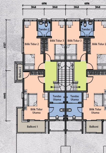
PELAN TINGKAT SATU UKURAN: 1:50
