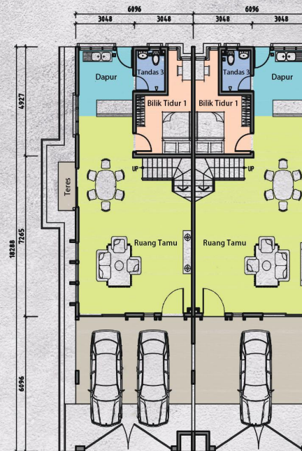
PELAN TINGKAT BAWAH UKURAN: 1:50
