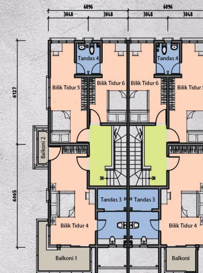
PELAN TINGKAT DUA UKURAN: 1:50
