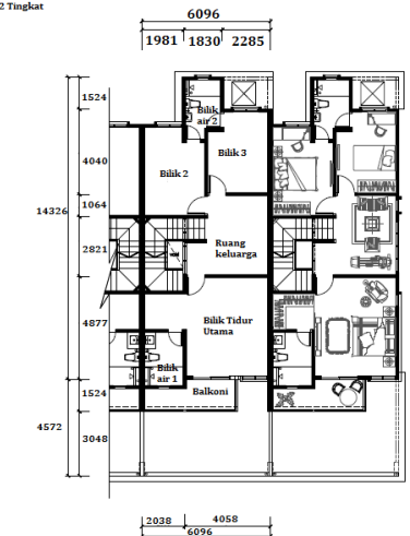
Rumah Teres 2 Tingkat Tingkat 1
