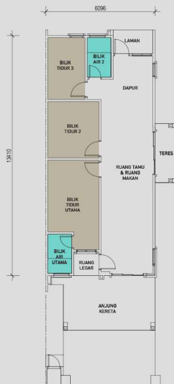
PELAN LANTAI
