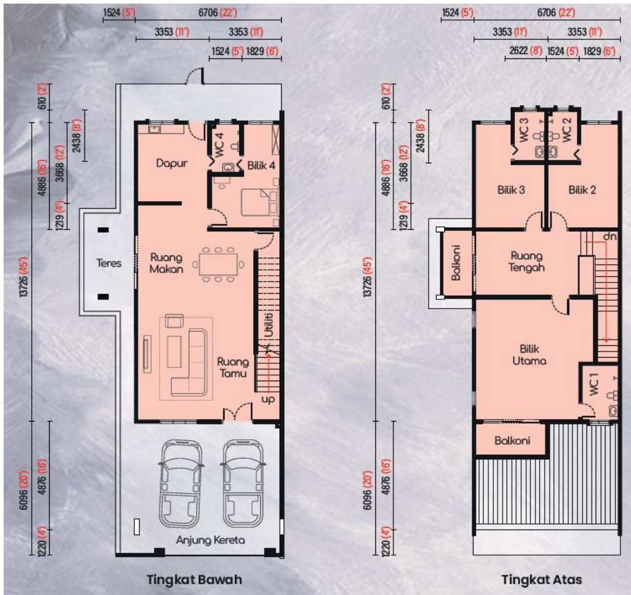
PELAN LANTAI JENIS B (LOT TEPI)
