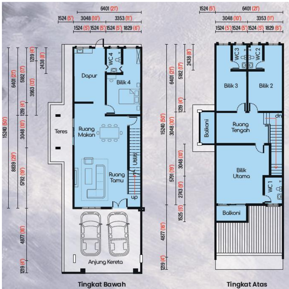
PELAN LANTAI JENIS A (LOT TEPI)
