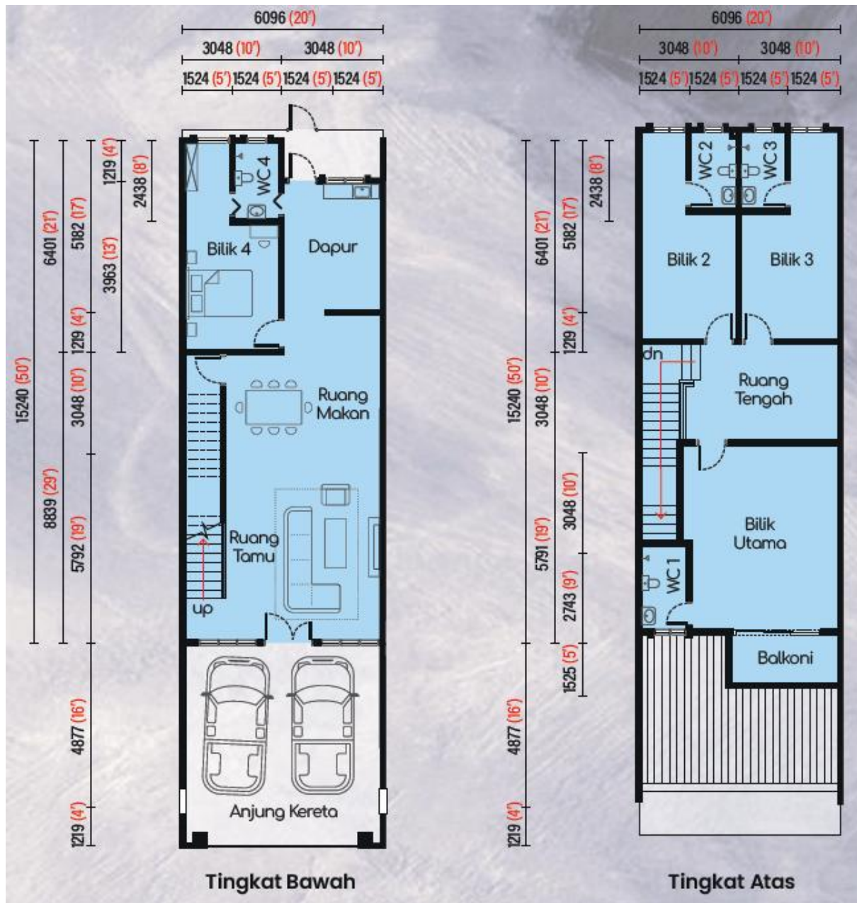
PELAN LANTAI JENIS A (LOT TENGAH)
