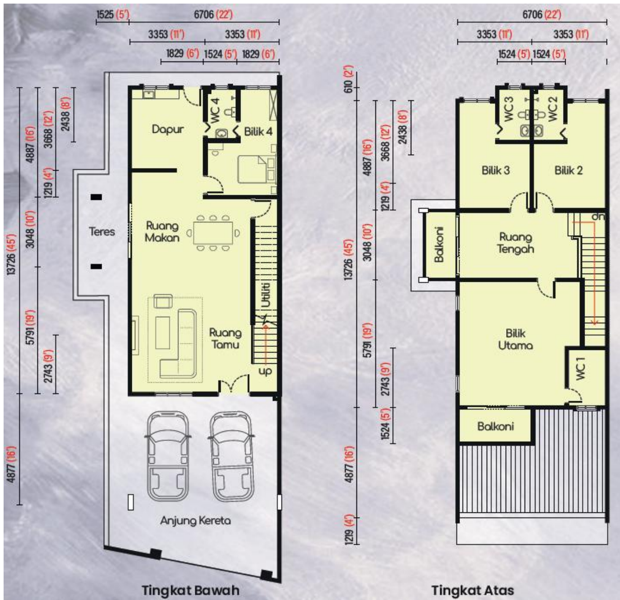
PELAN LANTAI JENIS C (LOT TEPI)
