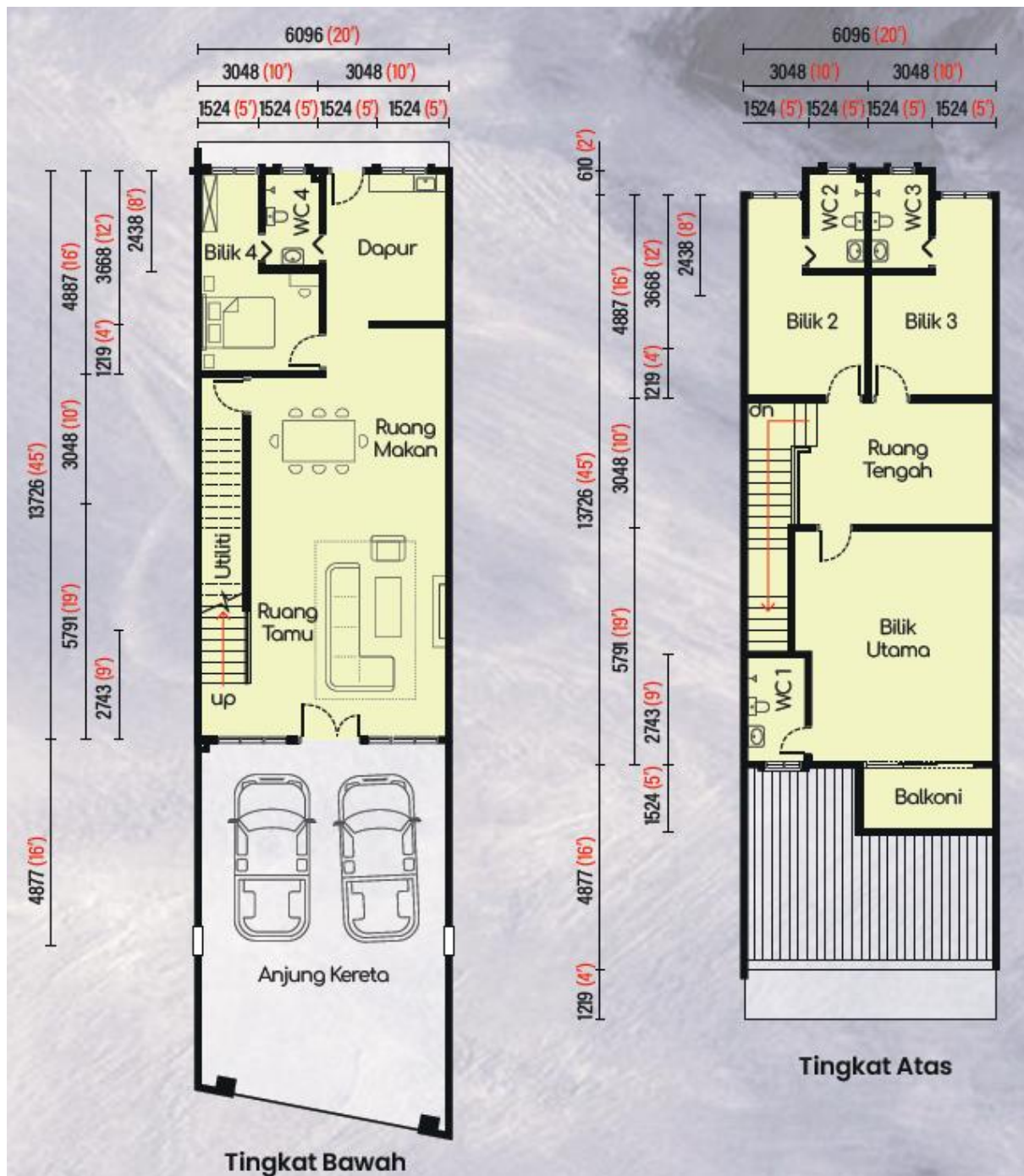
PELAN LANTAI JENIS C (LOT TENGAH)
