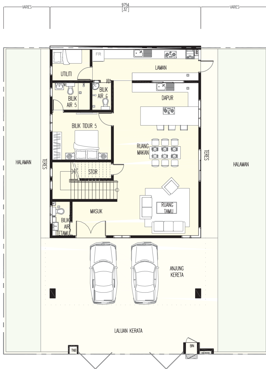
Jenis B1- Pelan Tingkat Bawah
