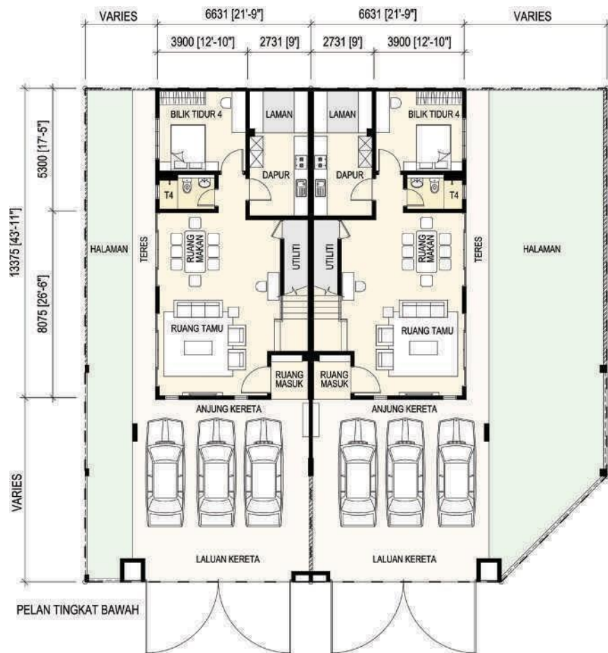
Jenis A1- Pelan Tingkat Bawah
