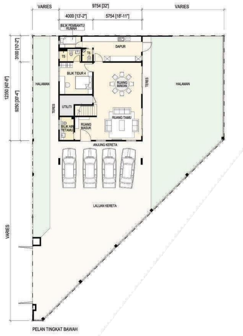
Jenis A3 - Pelan Tingkat Bawah
