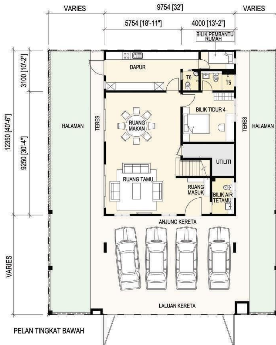
Jenis B2- Pelan Tingkat Bawah
