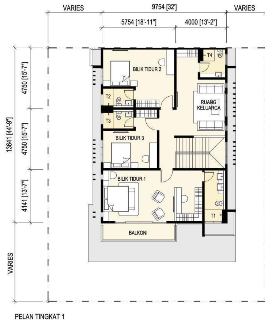
Jenis B2- Pelan Tingkat Pertama
