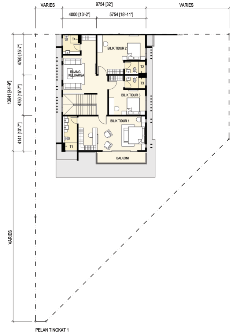
Jenis A3 - Pelan Tingkat Pertama
