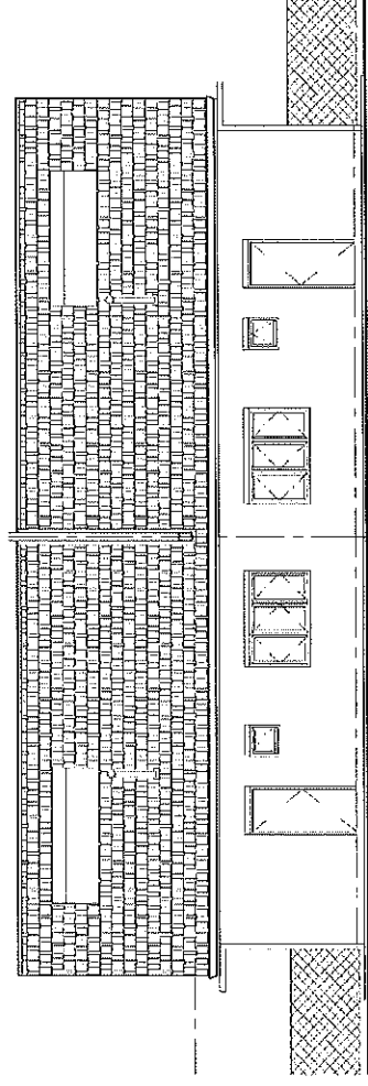
PANDANGAN BELAKANG
