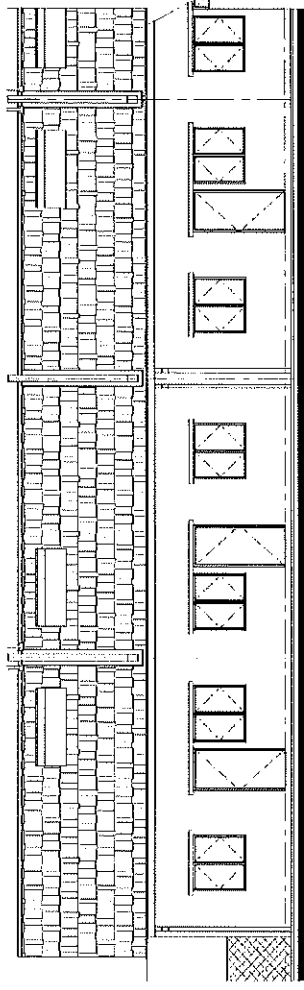
PANDANGAN BELAKANG
