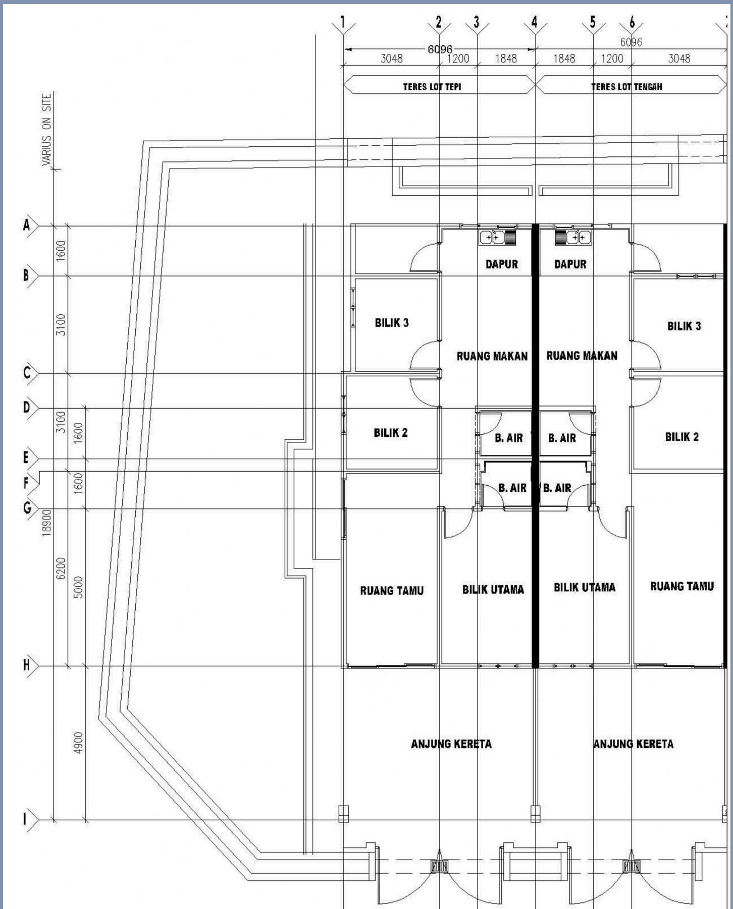
PELAN LANTAI RUMAH TERES
