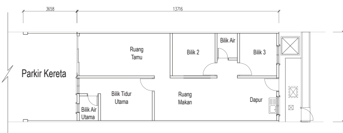
Pelan Lantai
