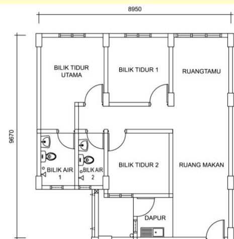
PELAN LANTAI 平面图
