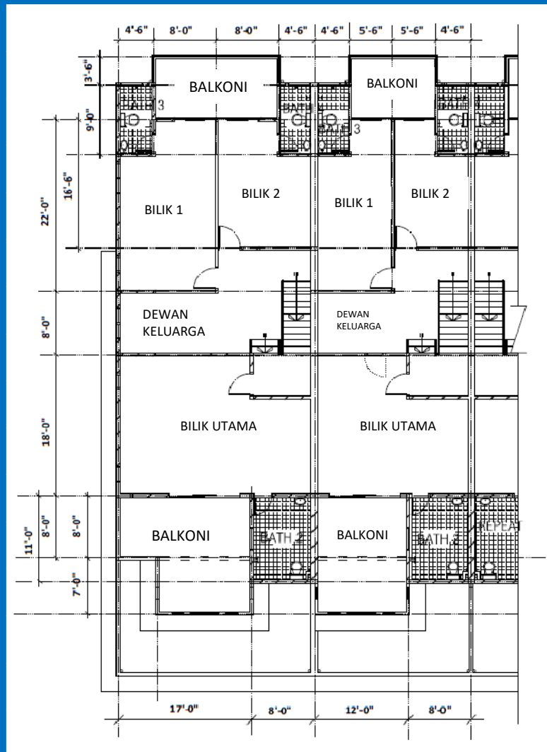
Pelan Tingkat Satu
