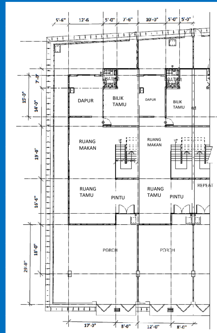
Pelan Tingkat Bawah
