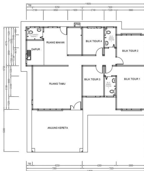
PELAN LANTAI
