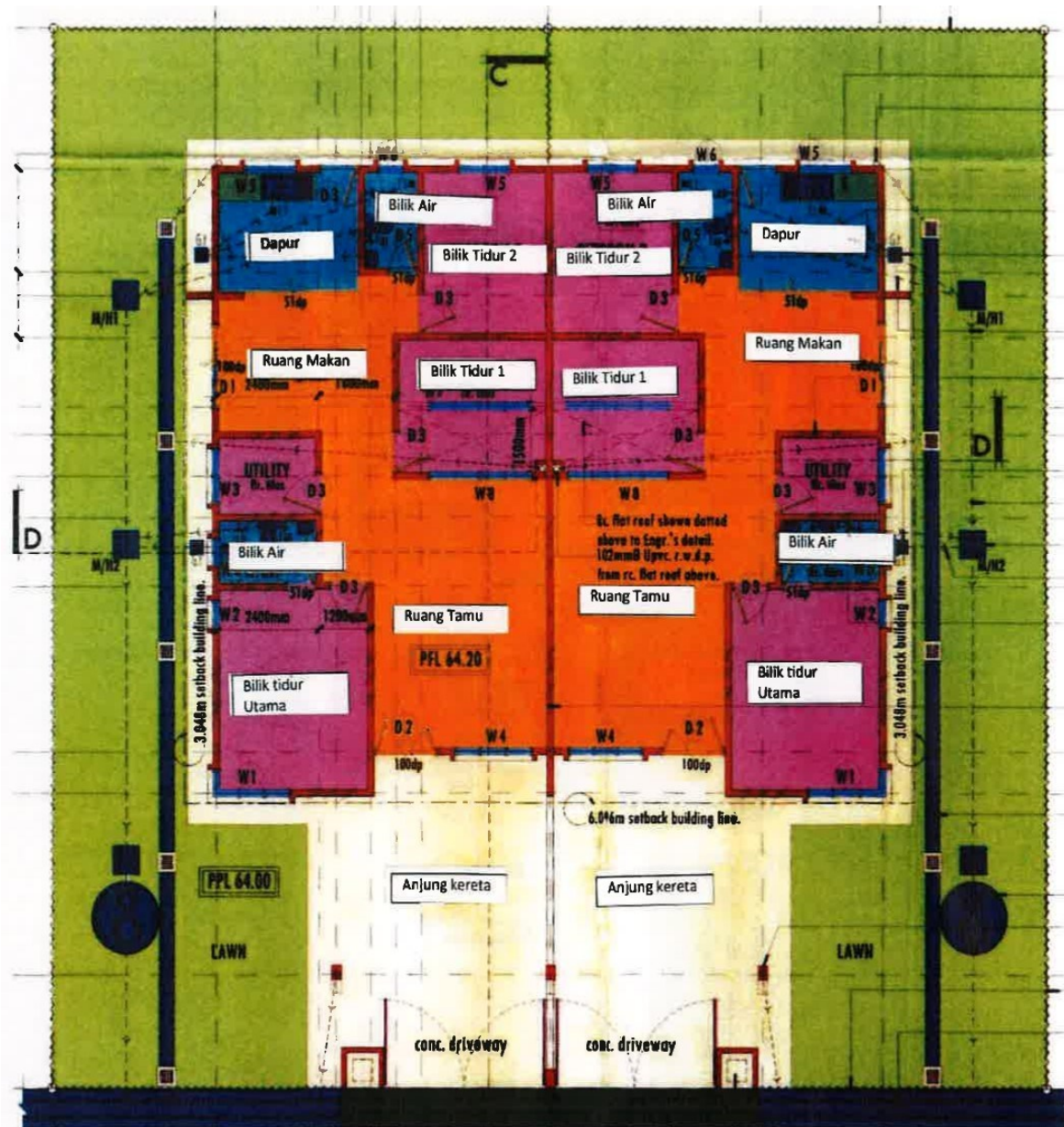
PELAN LANTAI
