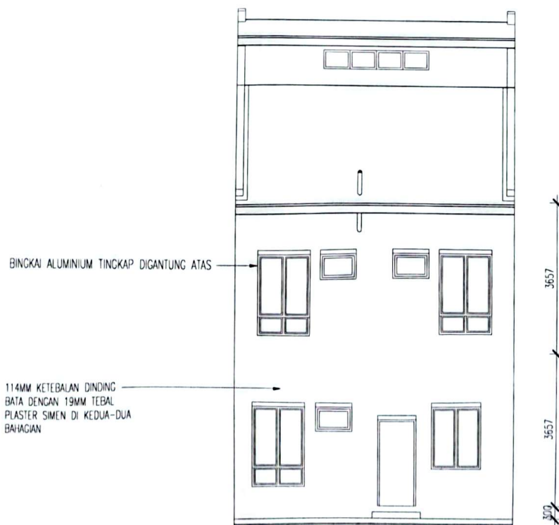
PANDANGAN BELAKANG
