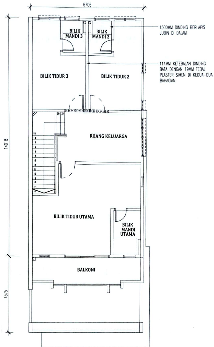
PELAN LANTAI SATU
