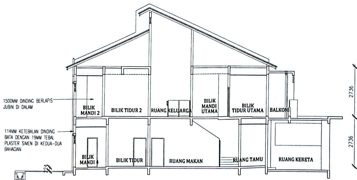
KERATAN
