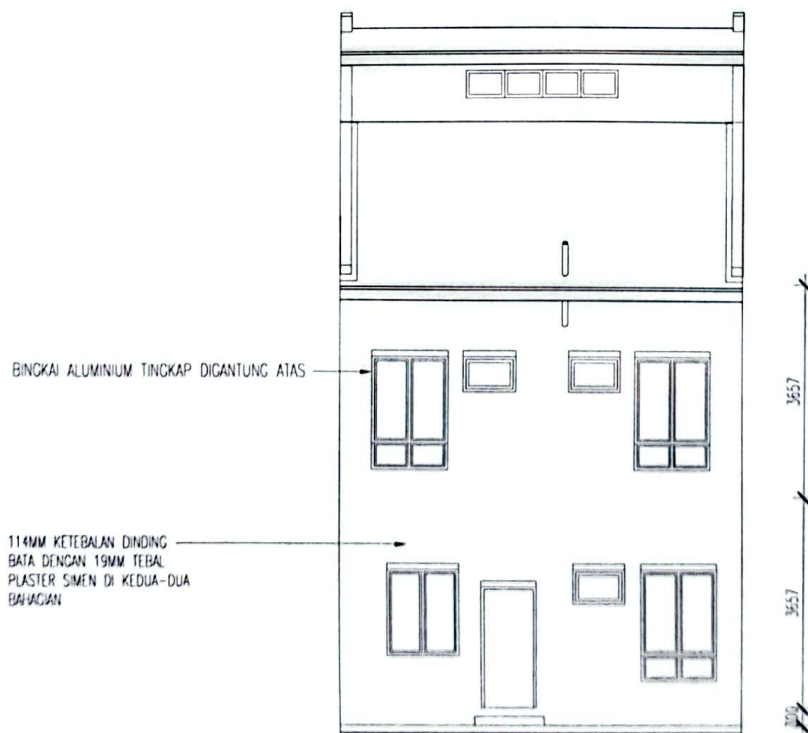
PANDANGAN BELAKANG
