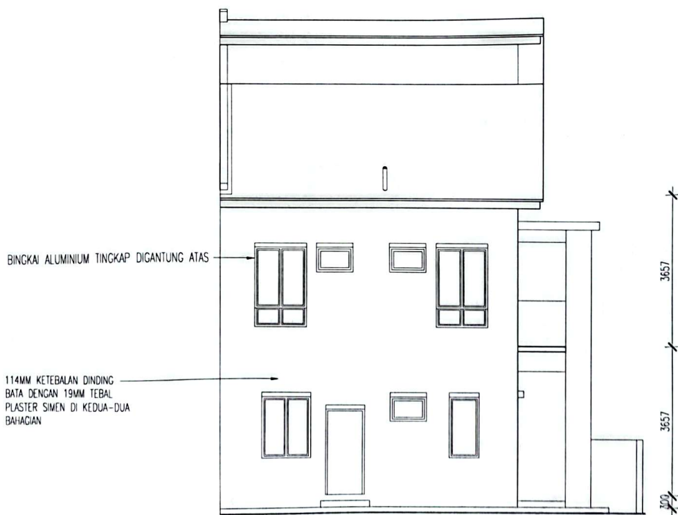
PANDANGAN BELAKANG
