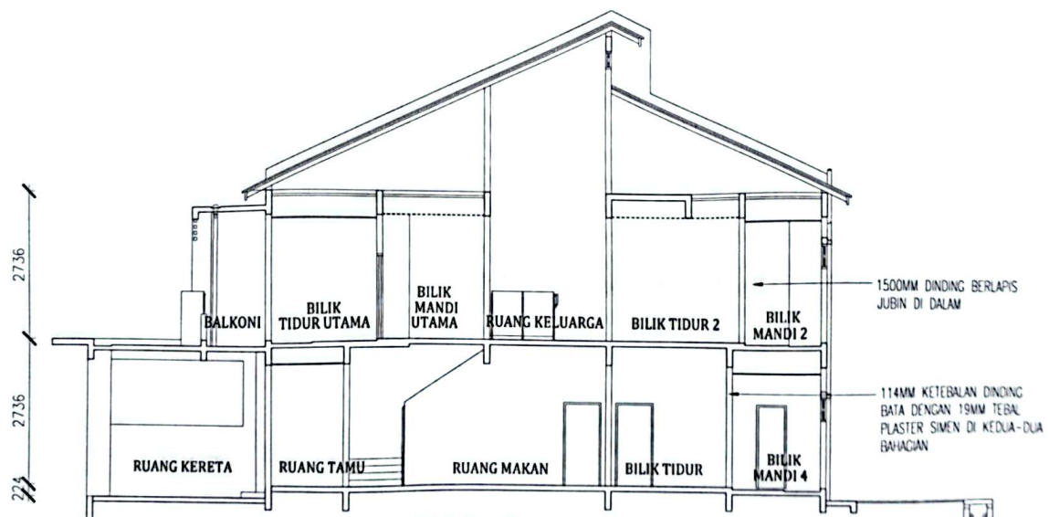
KERATAN
