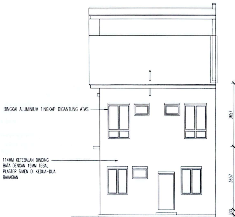
PANDANGAN BELAKANG
