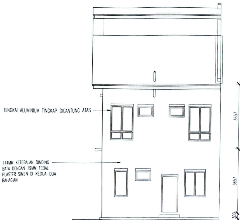
PANDANGAN BELAKANG
