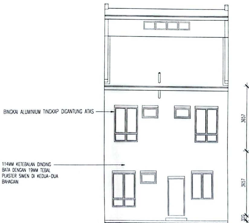
PANDANGAN BELAKANG
