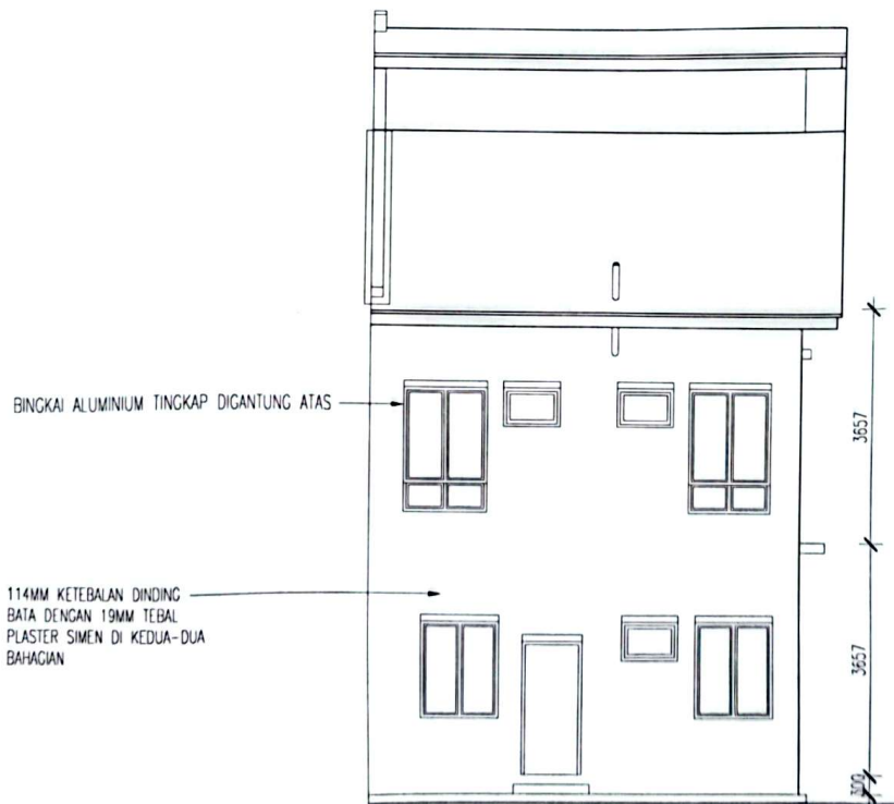
PANDANGAN BELAKANG
