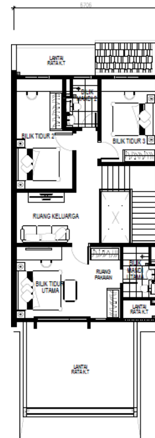
Pelan Lantai Rumah Teres 2 Tingkat Aras Satu
