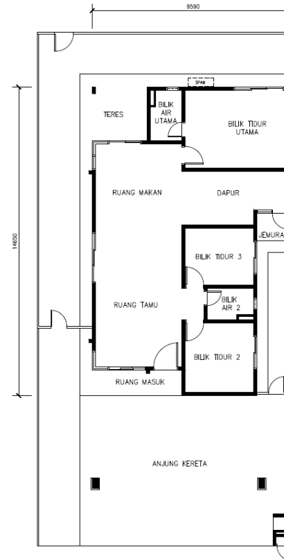
Pelan Lantai Rumah Berkembar 1-Tingkat
