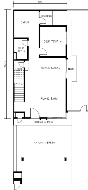
Pelan Lantai Rumah Klaster 2 Tingkat Aras Bawah
