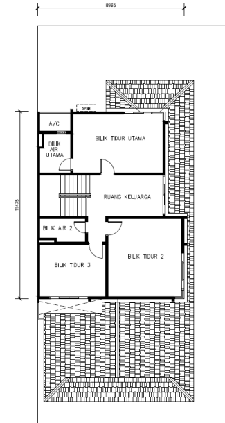
Pelan Lantai Rumah Berkembar 2 Tingkat Aras Satu
