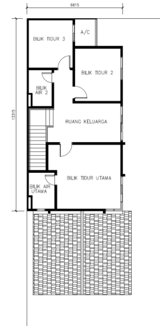
Pelan Lantai Rumah Klaster 2 Tingkat Aras Satu
