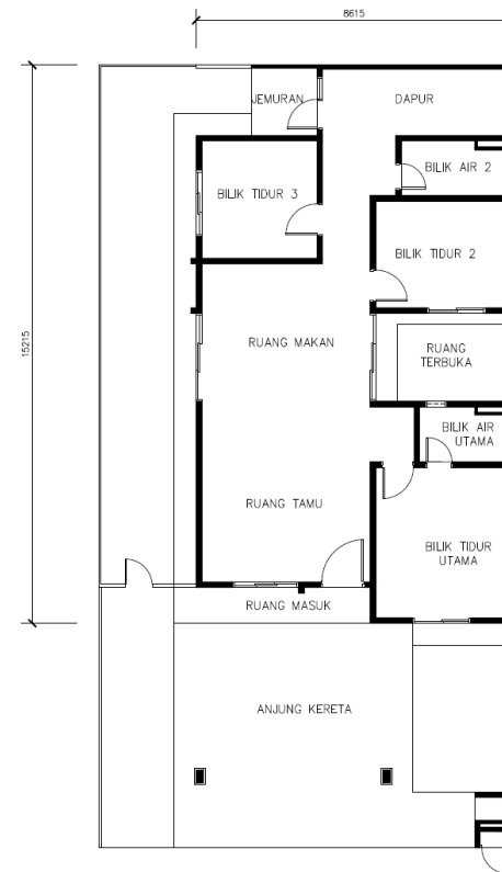
Pelan Lantai Rumah Klaster 1-Tingkat
