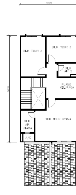
Pelan Lantai Rumah Teres 2 Tingkat Aras Satu
