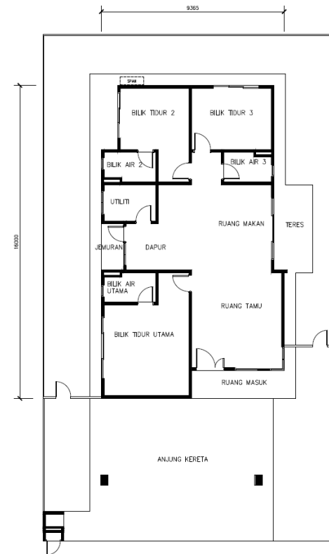
Pelan Lantai Rumah Sesebuah 1-Tingkat
