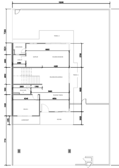
Pelan Lantai Rumah Berkembar 2 Tingkat Aras Bawah
