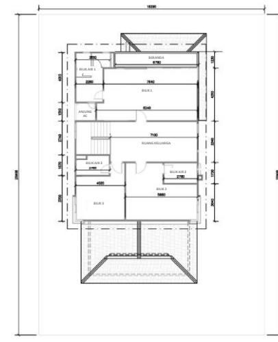
Pelan Lantai Rumah Sesebuah 2 Tingkat Aras Satu
