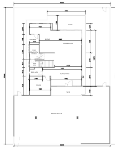
Pelan Lantai Rumah Sesebuah 2 Tingkat Aras Bawah
