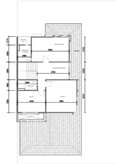
Pelan Lantai Rumah Berkembar 2 Tingkat Aras Satu
