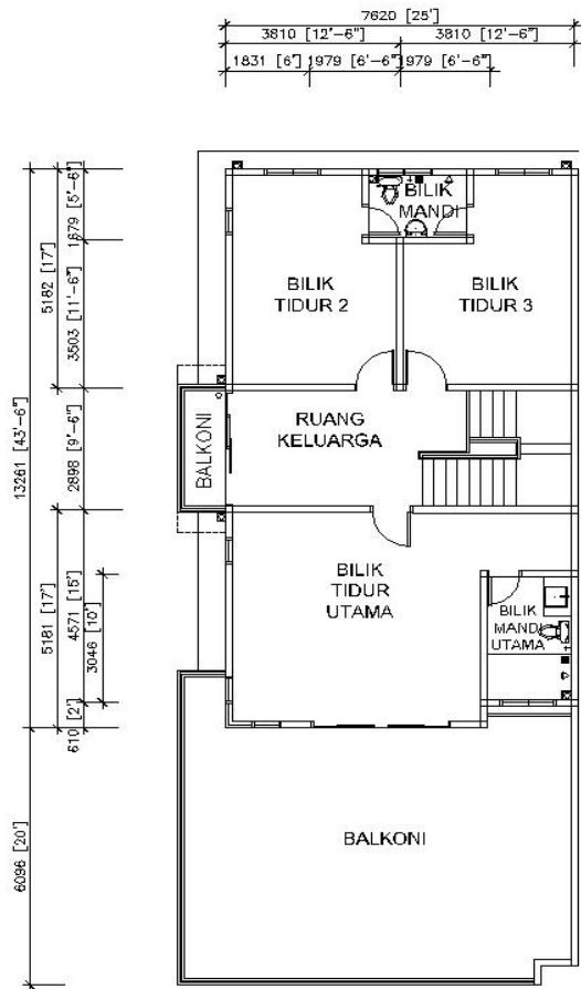
PELAN TINGKAT 1 SEMI-D JENIS A
