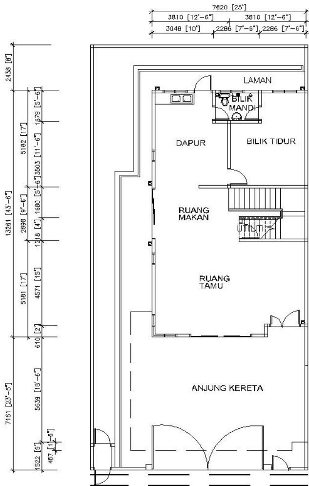
PELAN TINGKAT BAWAH SEMI-D JENIS A
