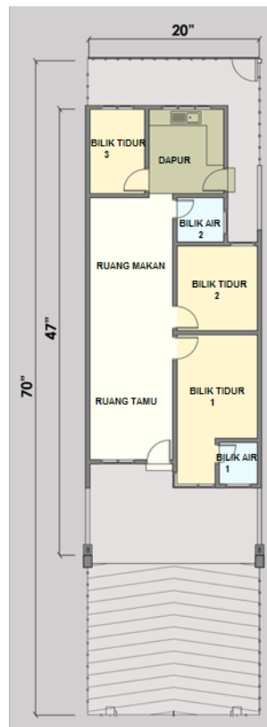
PELAN LANTAI
