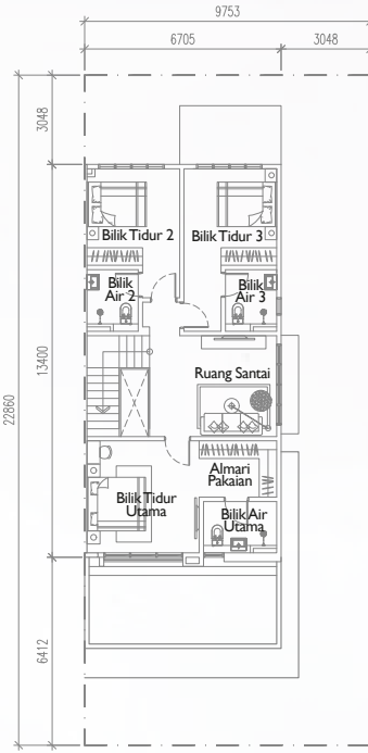
Tingkat Atas
