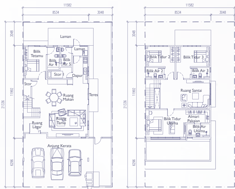
Tingkat Bawah
