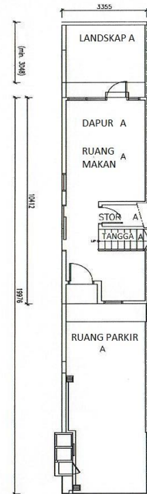
PELAN LANTAI TINGKAT BAWAH
