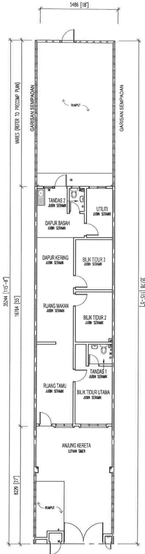
PELAN LANTAI
