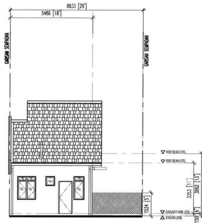
PANDANGAN BELAKANG
