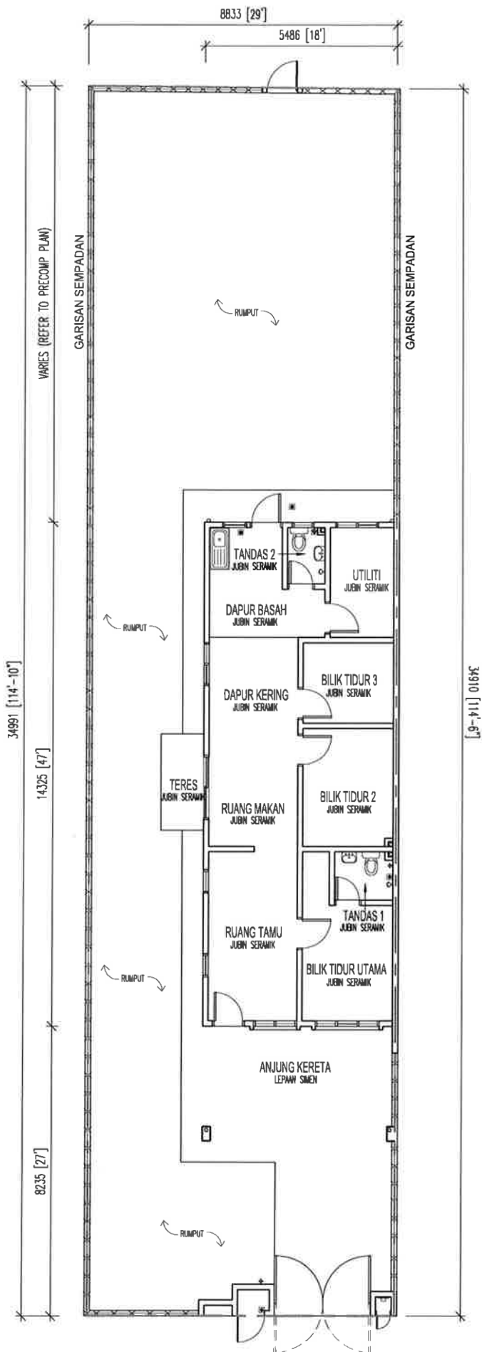
PELAN LANTAI
