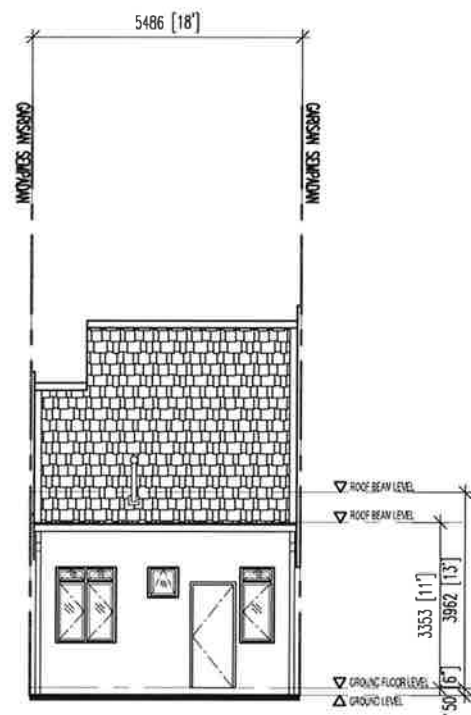
PANDANGAN BELAKANG
