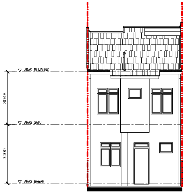
PANDANGAN BELAKANG
