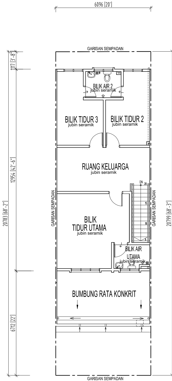
PELAN LANTAI TINGKAT SATU
