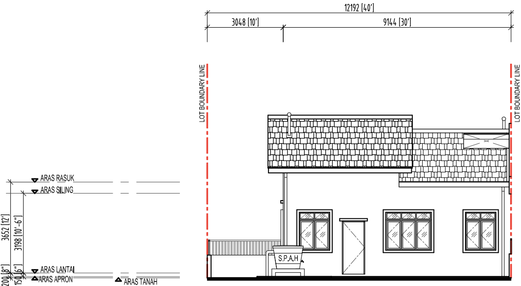
PANDANGAN BELAKANG
