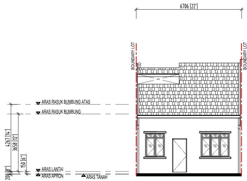
PANDANGAN BELAKANG
