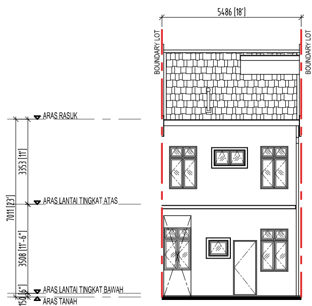
PANDANGAN BELAKANG
