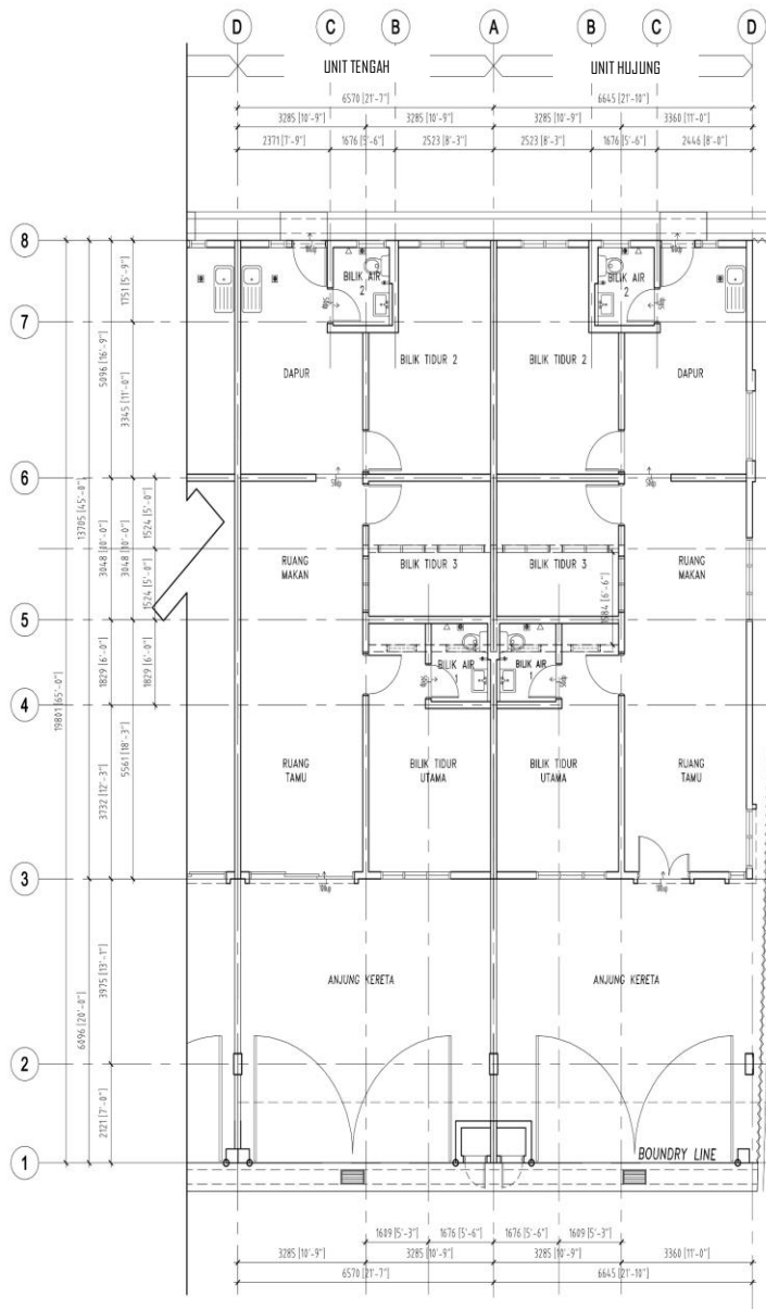
PELAN LANTAI
