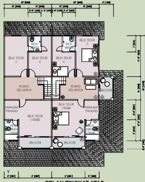
PELAN TINGKAT ATAS
