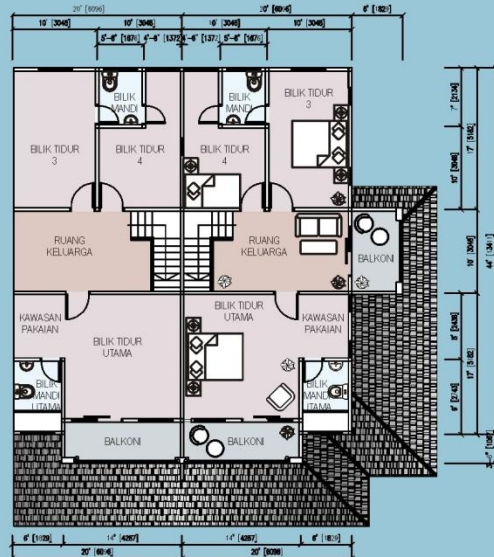
PELAN TINGKAT ATAS
