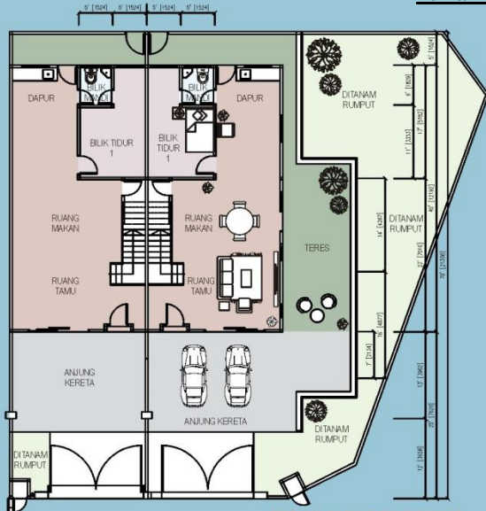
PELAN TINGKAT BAWAH
