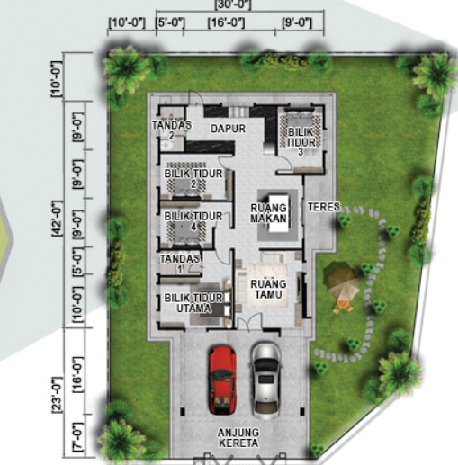
PELAN LANTAI RUMAH SESEBUAH JENIS "B"
