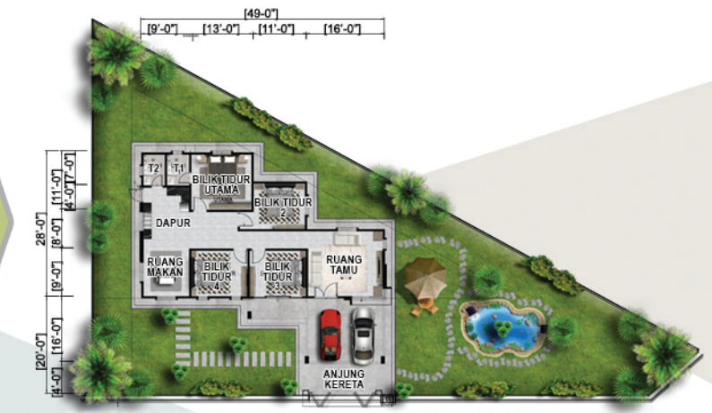
PELAN LANTAI RUMAH SESEBUAH JENIS "A"
